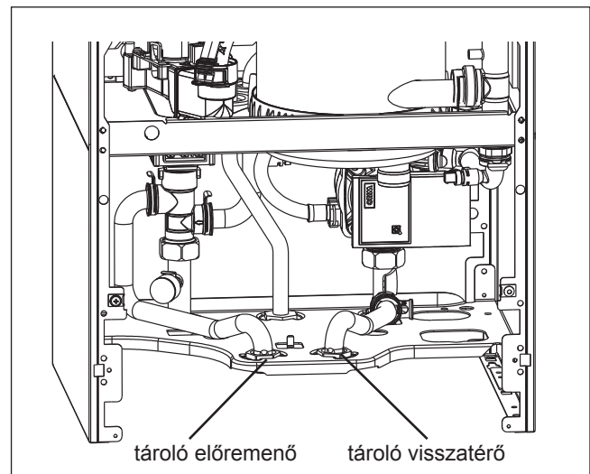
Ábra: A csatlakoztató blokk leszerelése
