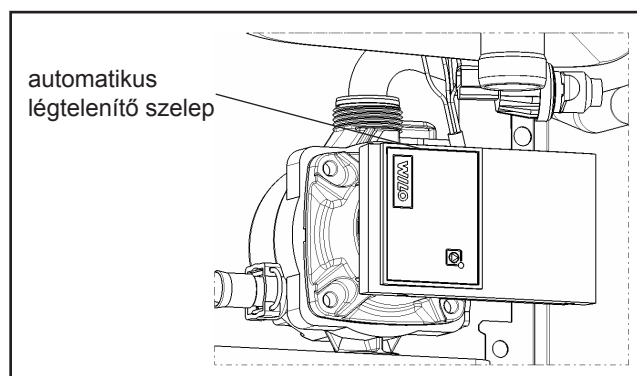
Ábra: Automatikus légtelenítő szelep a fűtőköri szivattyún
