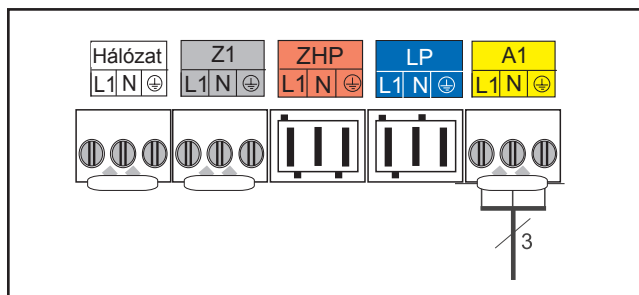
Ábra: A1-es csatl. kimenet
