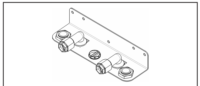
Ábra: Beépítő konzol vakolat feletti szereléshez (tartozékként vásárolható) a CGB-2K falikazánhoz
