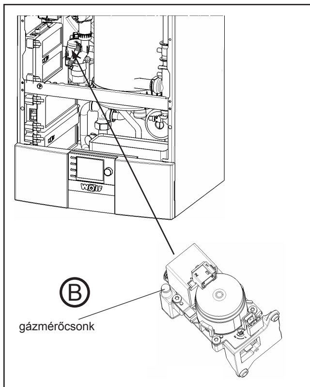
Ábra: A gáznyomás mérése
