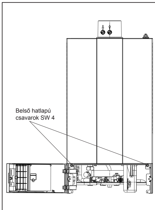
Ábra: Előlnézet – a szabályozó fedele teljesen kinyitva
