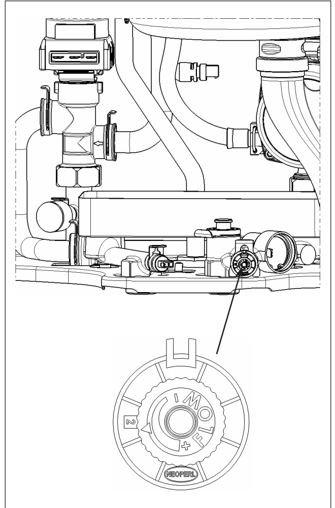
Ábra: A HMV-mennyiség beállítása
