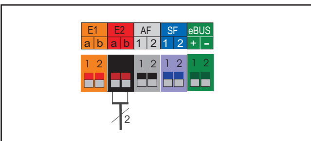
Ábra: Az E2 bemenet csatlakoztatása
