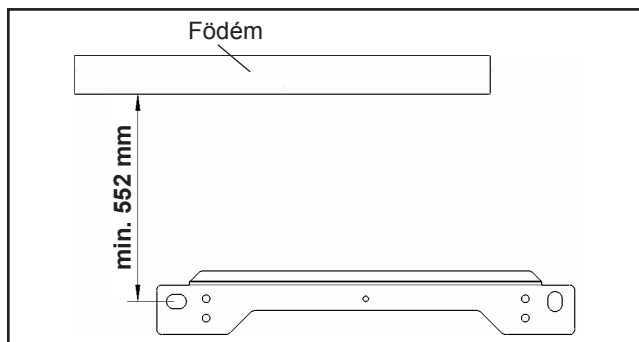
Ábra: A felasztó váll furatai
