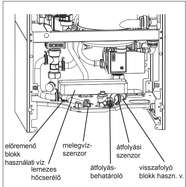
Ábra: A kombi kazán csővezetékei
