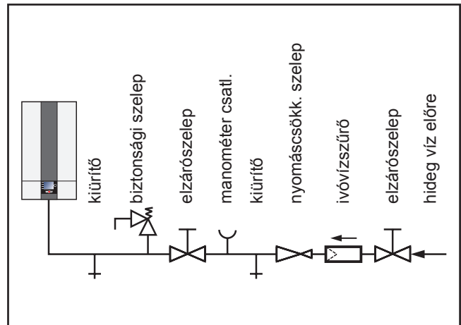
Ábra: Hidegvíz-csatlakozás
