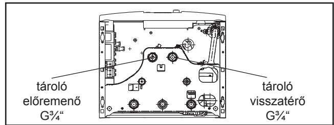
Ábra: HMV-tároló előremenő- és visszatérő csatlakozó
