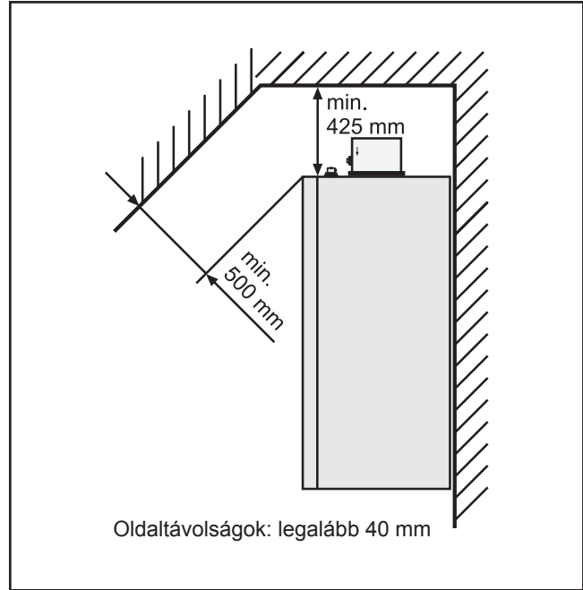
Ábra: A minimális telepítési távolságok
