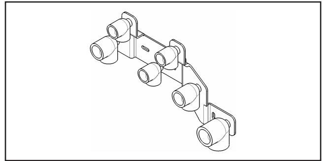
Ábra: Beépítő konzol vakolat alatti szereléshez (tartozékként vásárolható) a CGB-2K falikazánhoz
