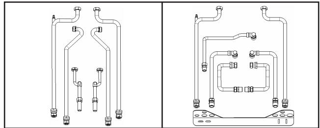
Ábra: Csatlakozókészlet Wolf tárolóhoz, CSW-120 típus, vakolat alatti szereléshez (tartozékként vásárolható)
