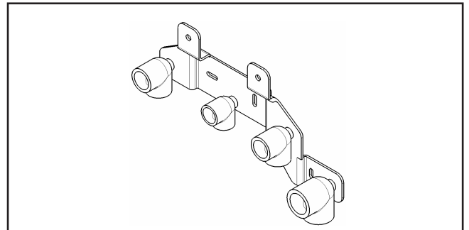
Ábra: Beépítő konzol vakolat alatti szereléshez (tartozékként vásárolható) a CGB-2 falikazánhoz
