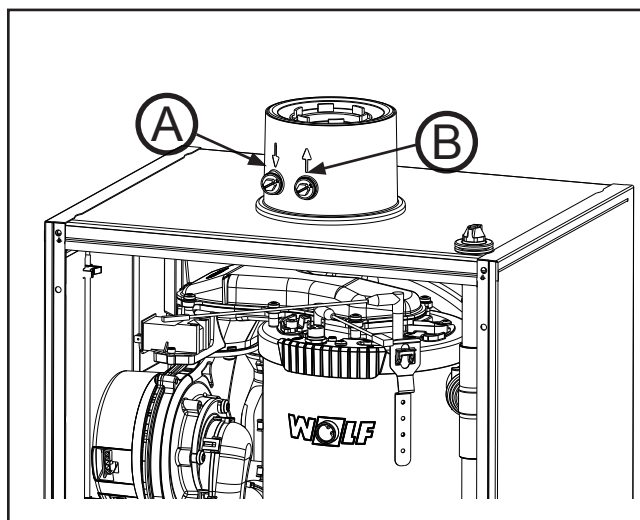
Ábra: A füstgáz paraméterek mérése
