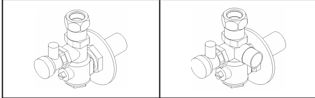
Ábra: Sarok elzárócsap ürítőcsappal (tartozékként vásárolható)
